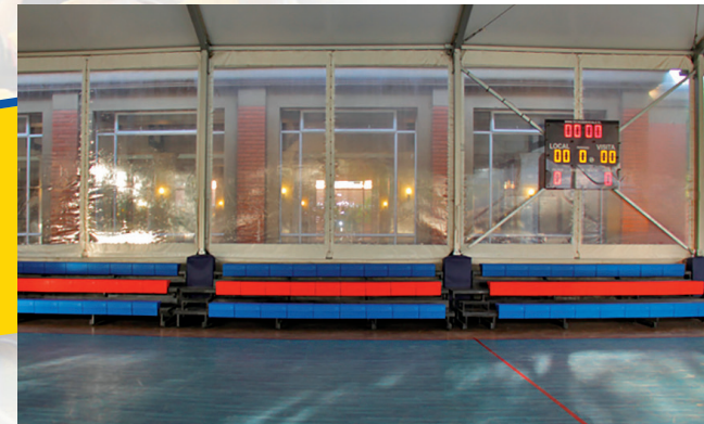
Galerías retráctiles para el gimnasio del Colegio Tabancura.
